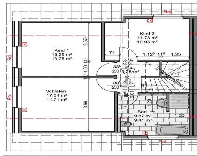
Dachgeschoss
